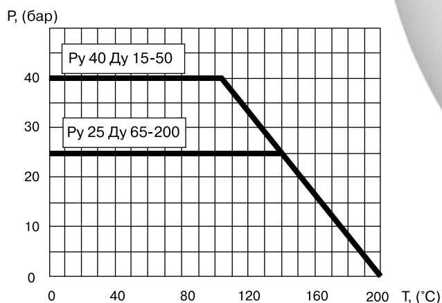
Зависимость «Температура-Давление»
